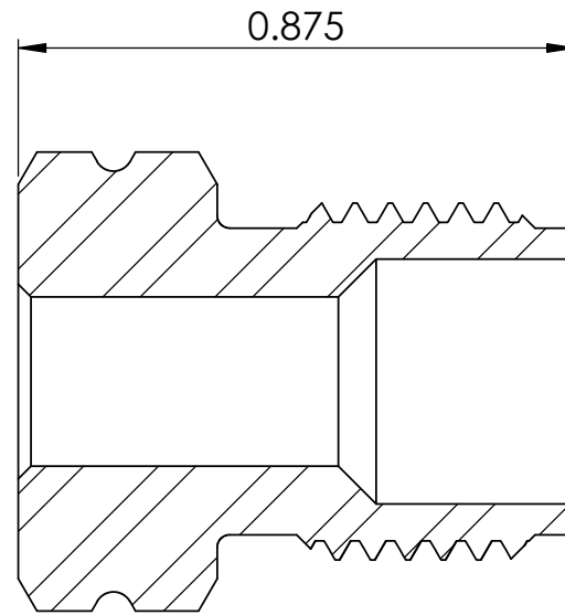
SECTION A-A SCALE 3 : 1
